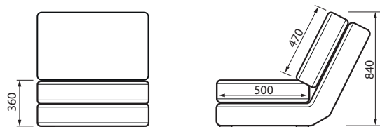
СЕКЦИЯ ОДНОМЕСТНАЯ 10
