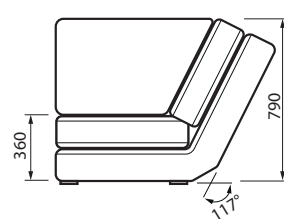
СЕКЦИЯ УГЛОВАЯ 90
